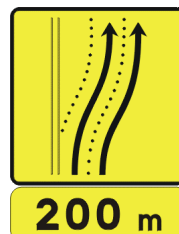
Panneau KD8 + panonceau KM1 – exemple 6
